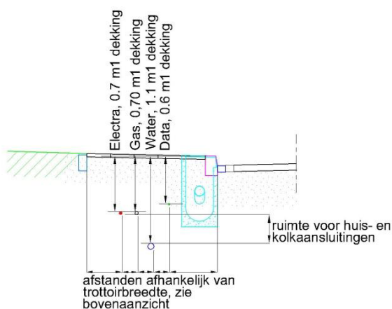
Doorsnede schaal 1:50
