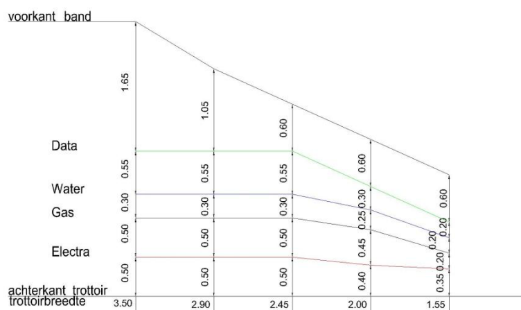
Bovenaanzicht schaal 1:50
