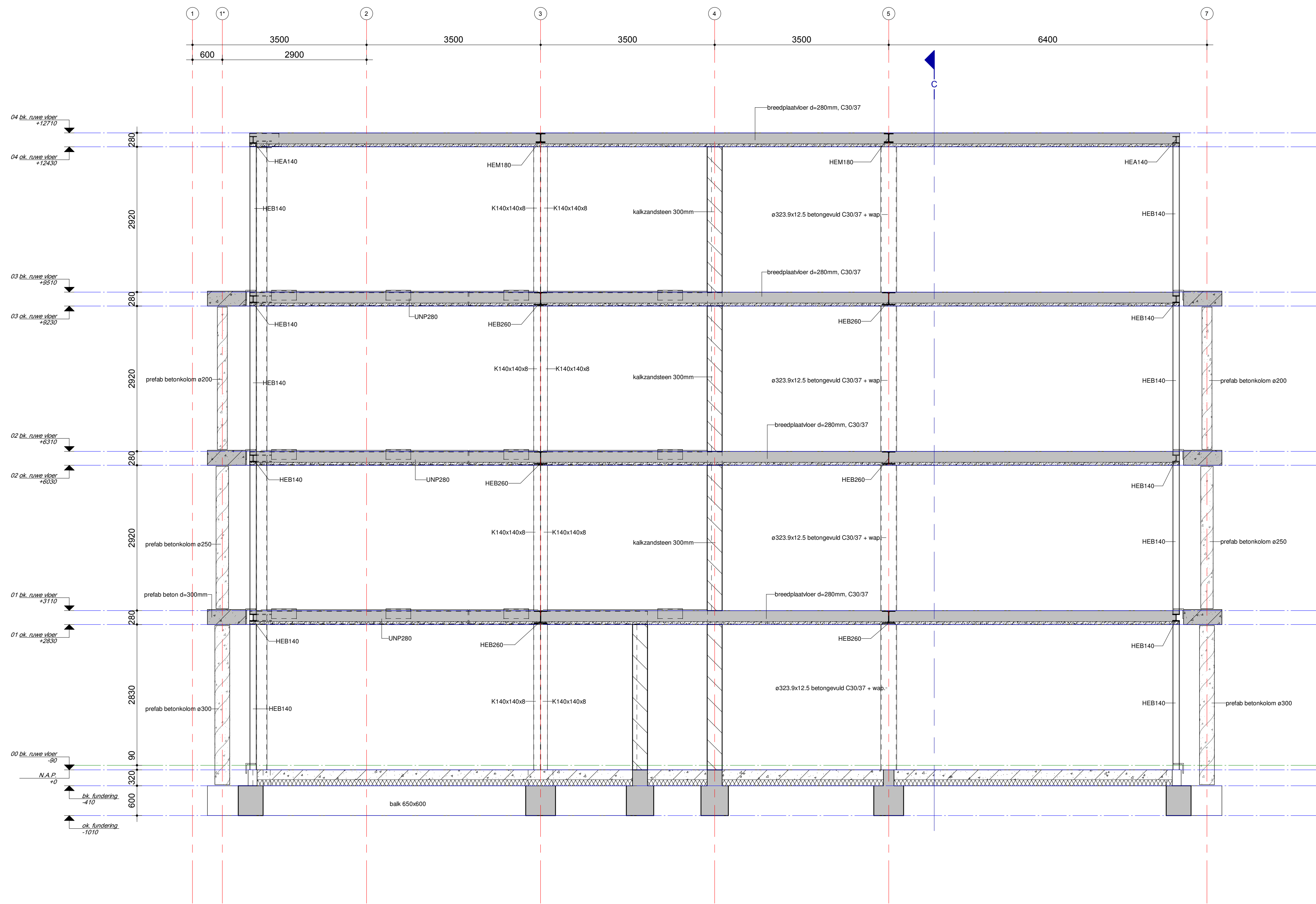
Doorsnede A 1 : 50
