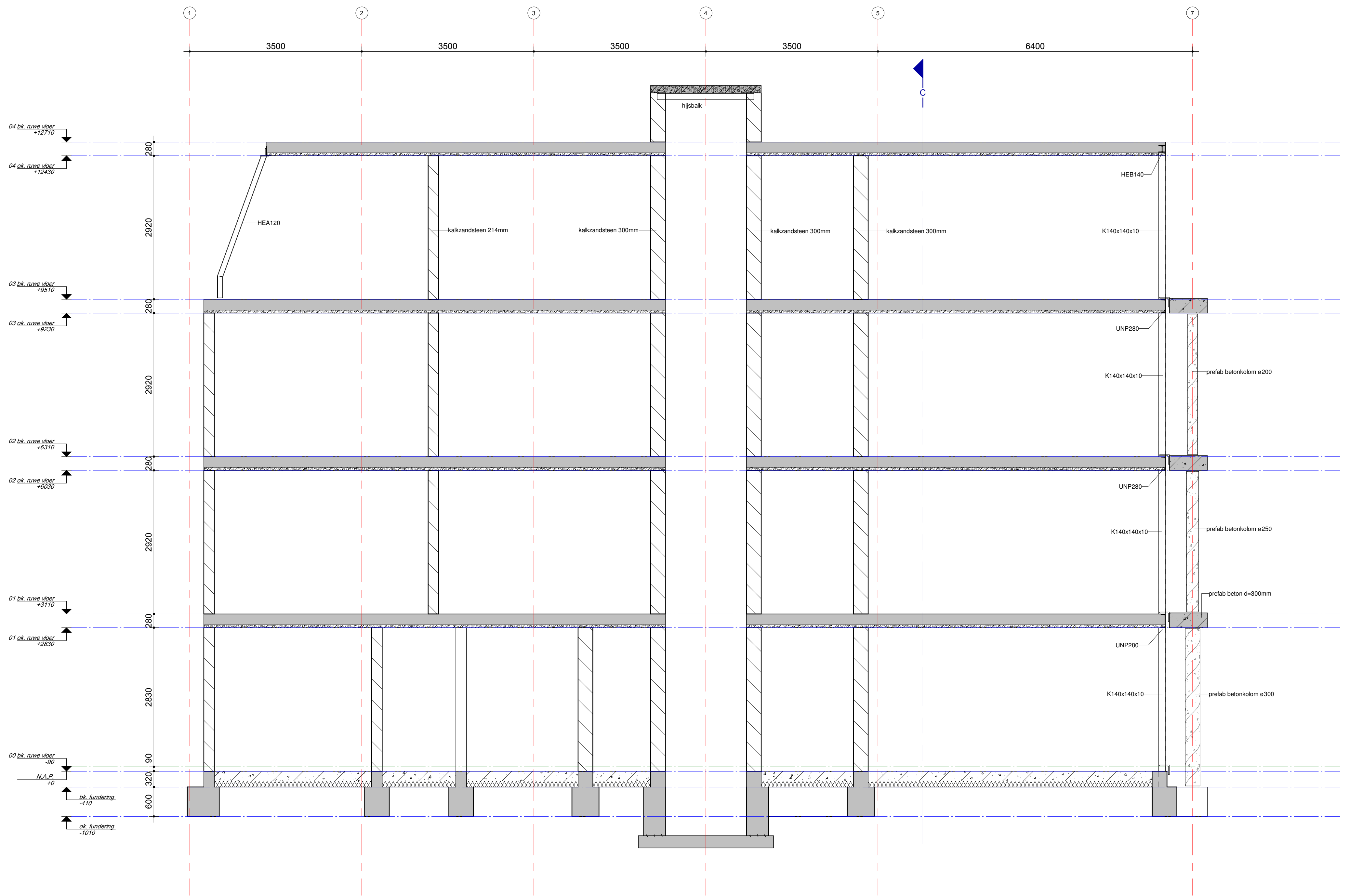
doorsnede B 1 : 50
