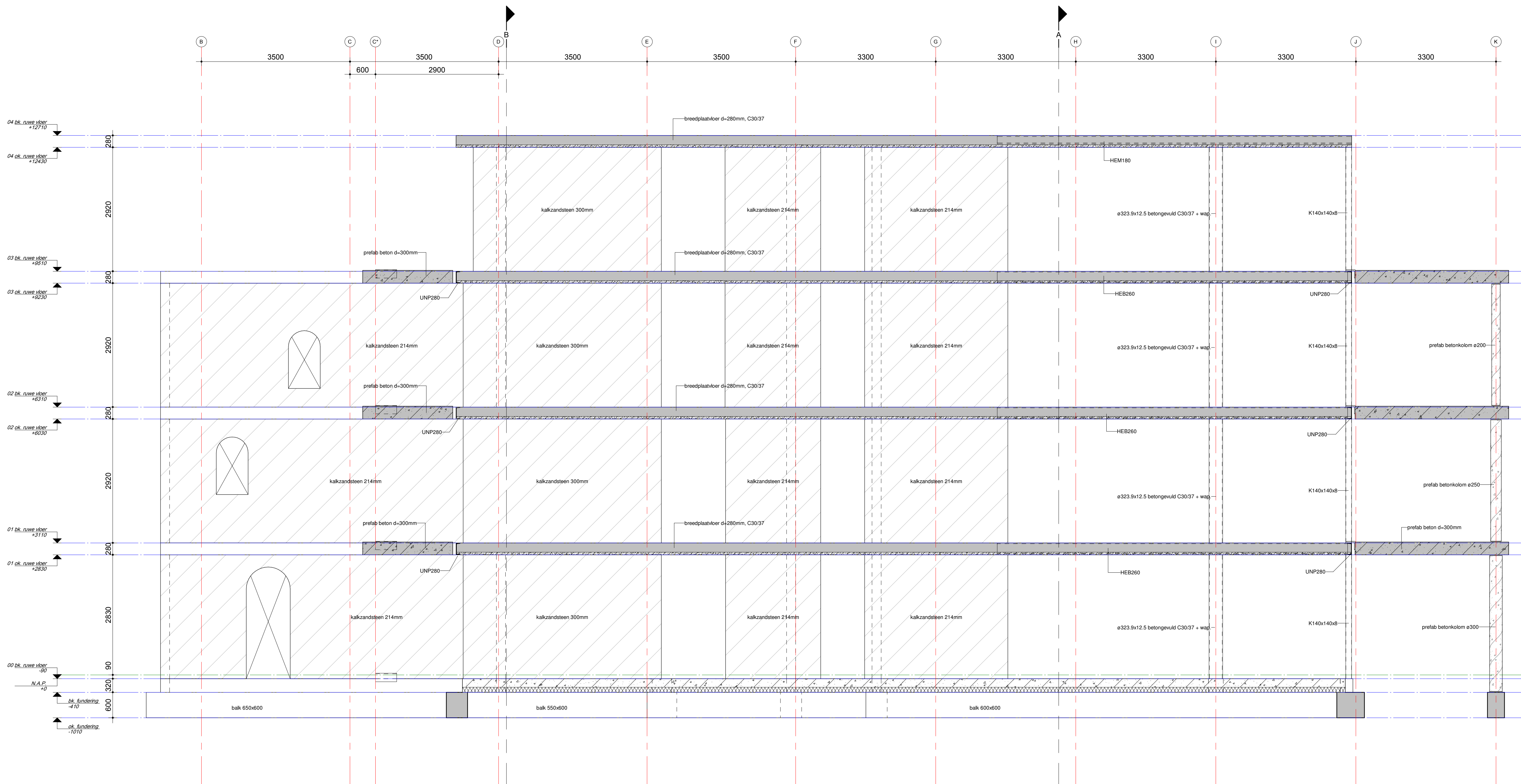
Doorsnede C 1 : 50
